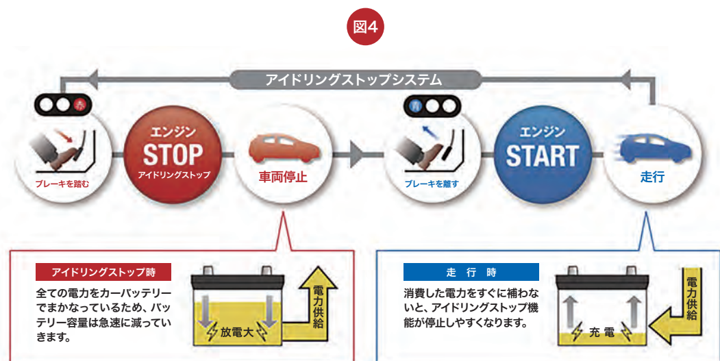
一時停車時にエンジンを停止し、燃料の消費を抑える仕組み
