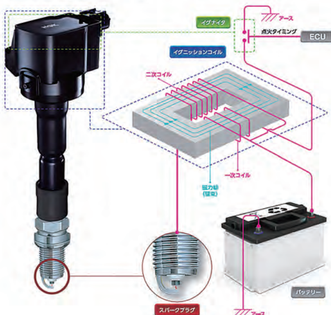
【一般的なイグニッションコイルの接続回路図】
