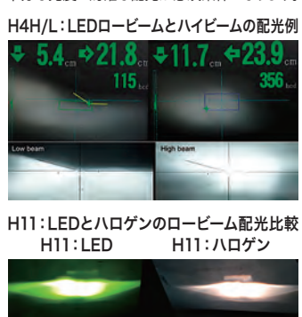
ヘッドライトテスターにおける光度と光軸検査例
