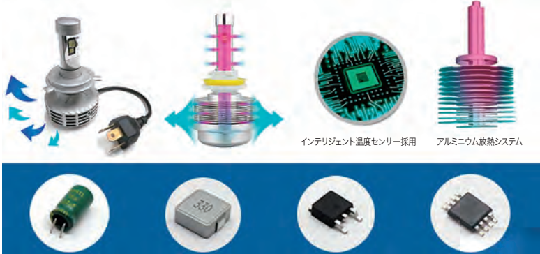
LED製品の様々な放熱システムと制御装置について
