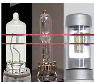
ハロゲン HID LED 発光原理は異なりますが、発光点を統一することにより、正確な配光、照射範囲を可能にしています。
