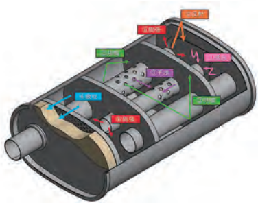
図④ 消音の原理
