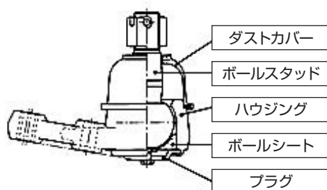
ボールジョイントの部品構成
